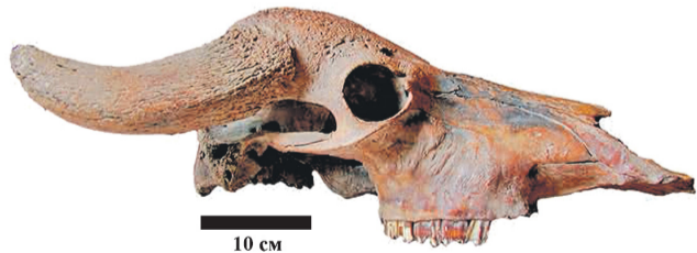
Череп европейского водяного буйвола. Четвертичный период (плейстоцен), берег реки Коломенки у села Лукерьино
