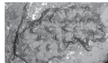
Колония мшанки. Юрский период, Коломенский щебеночный карьер
